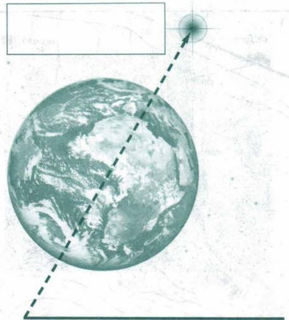
Плоскость орбиты Земли
