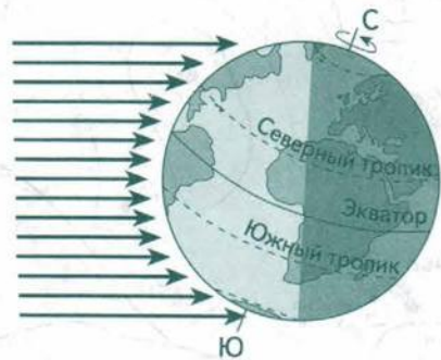
Плоскость орбиты Земли
